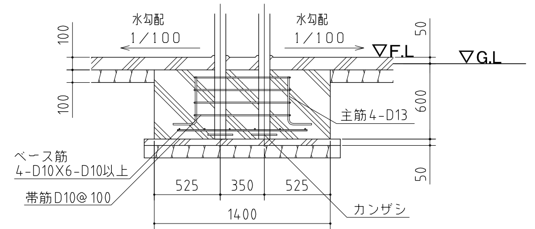
A-A' 断面
